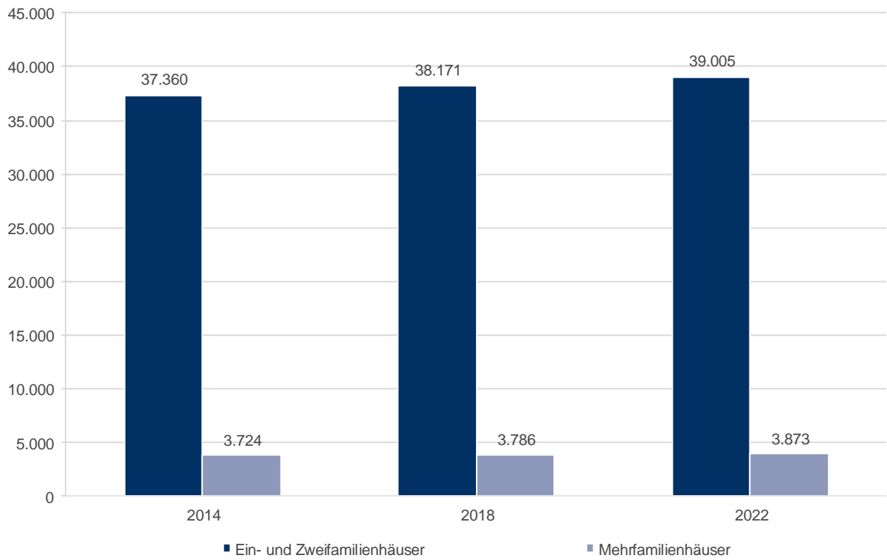
Abb. 11 | Wohngebäudebestand
